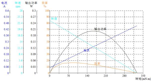
Model: WL-16RS03000611500-515K
