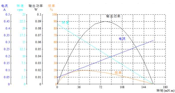
Model: WL-16RS0300036500-315K
