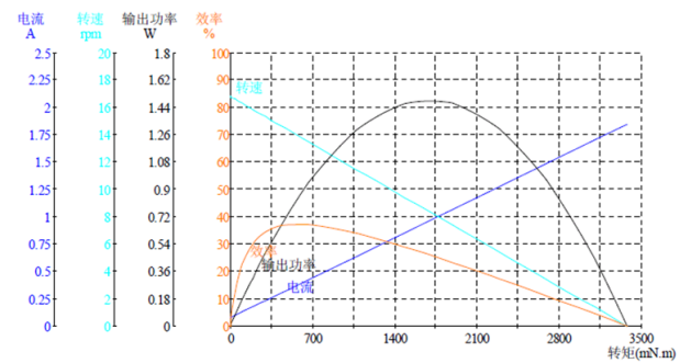
Model: WL-37RS5280064500-270K
