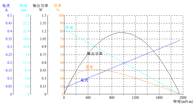
Model: WL-37RS5280244500-184K
