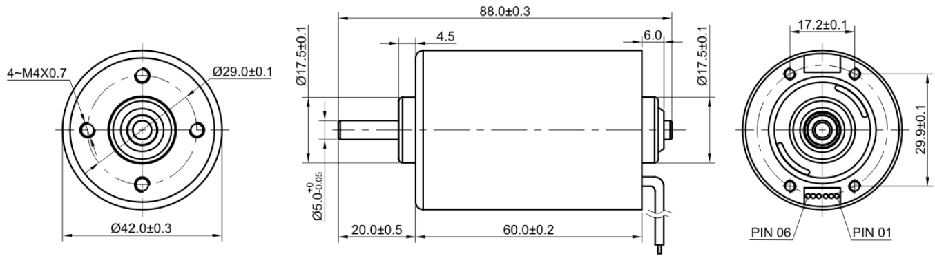
电机参数/ Motor Data :
